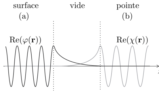
FIGURE 3: Dans son modèle, J. Bardeen considère des transitions électroniques possibles entre des états distincts des deux milieux (a) et (b).
