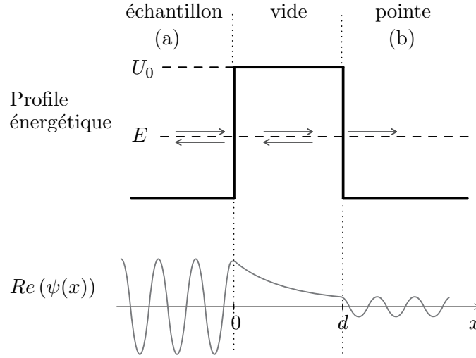
FIGURE 1: La jonction tunnel peut être modélisée en première approche par une barrière de potentiel quantique carrée. Le profil de la barrière est représenté, accompagné des différentes notations, ainsi que l'aspect de la partie réelle de l'amplitude de probabilité de présence d'un électron. L'état quantique peut se décomposer en plusieurs ondes transmises et réfléchies dans chacun des trois milieux (ce que représentent les cinq flèches).
